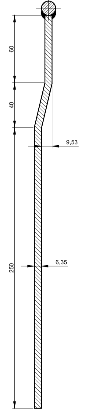
SECCION G-G ESCALA: 1:2
