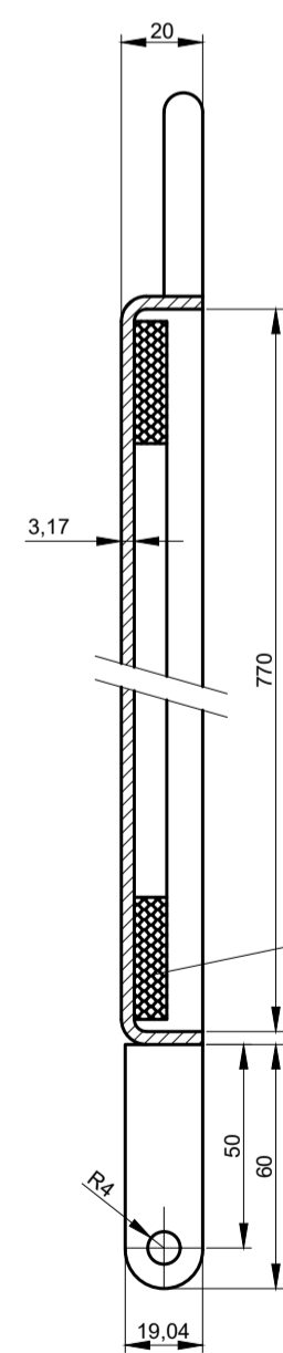
CORTE D-D ESCALA: 1:2
