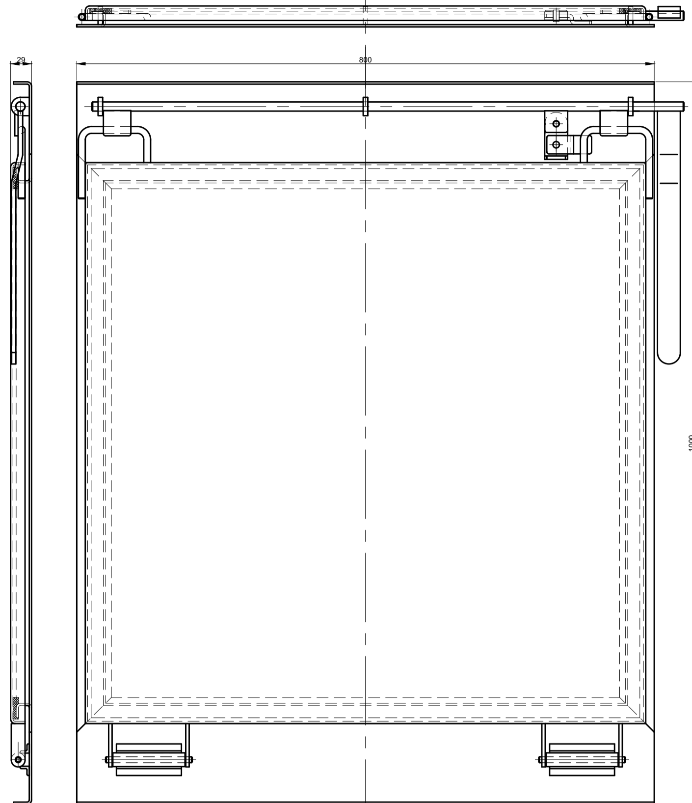
ESCOTILLA DE CARGA ESCALA: 1:5
