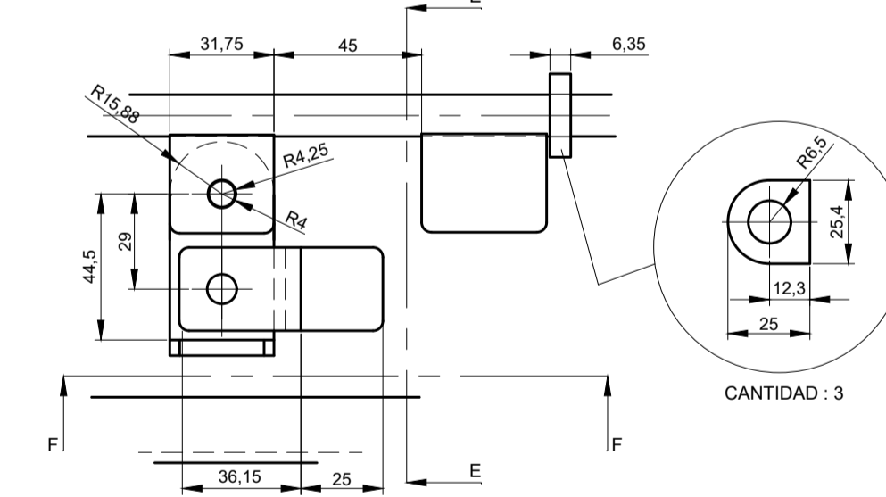
DETALLE A ESCALA: 1:2
