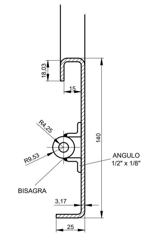
CORTE B-B ESCALA: 1:2
