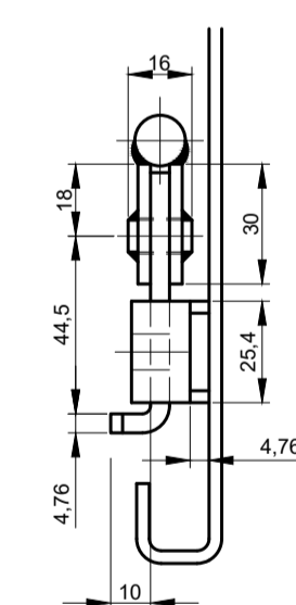
VISTA E-E ESCALA: 1:2
