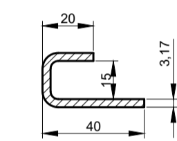
SECCION A-A ESCALA: 1:2
