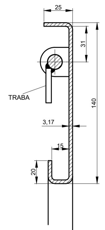
CORTE C-C ESCALA: 1:2
