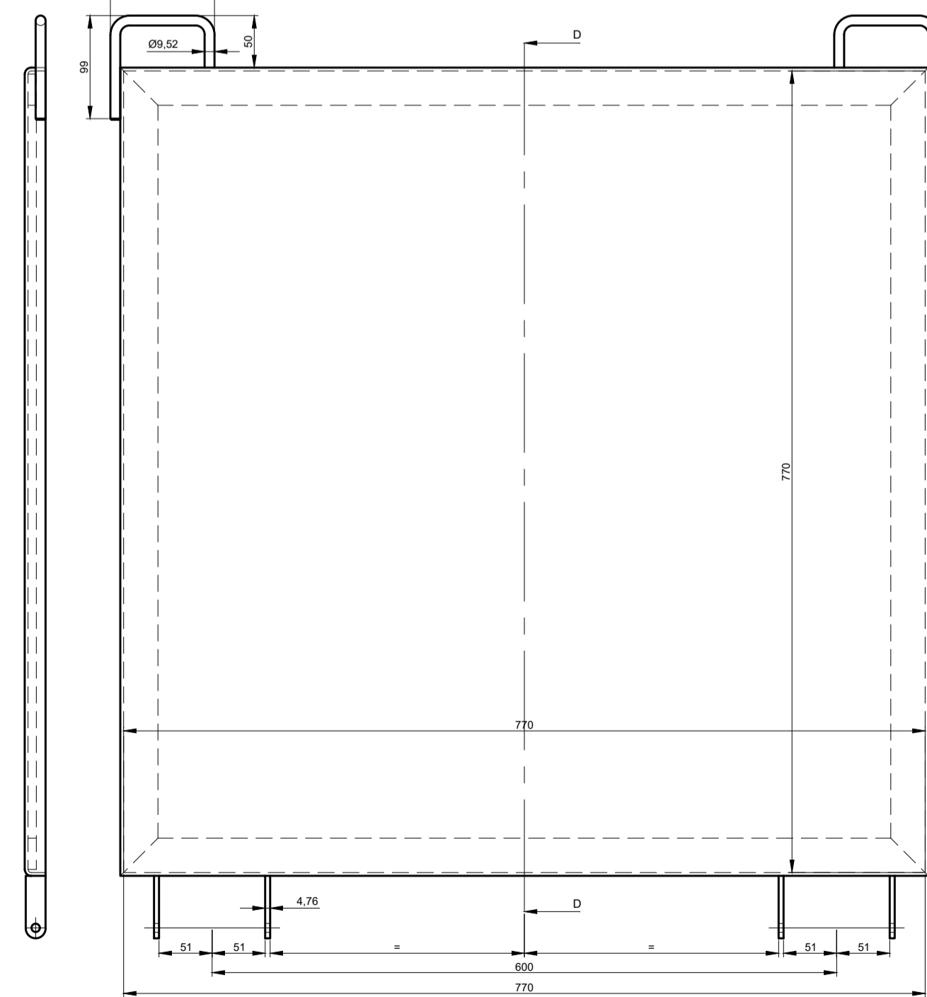
TAPA ESCOTILLA ESCALA: 1:5
