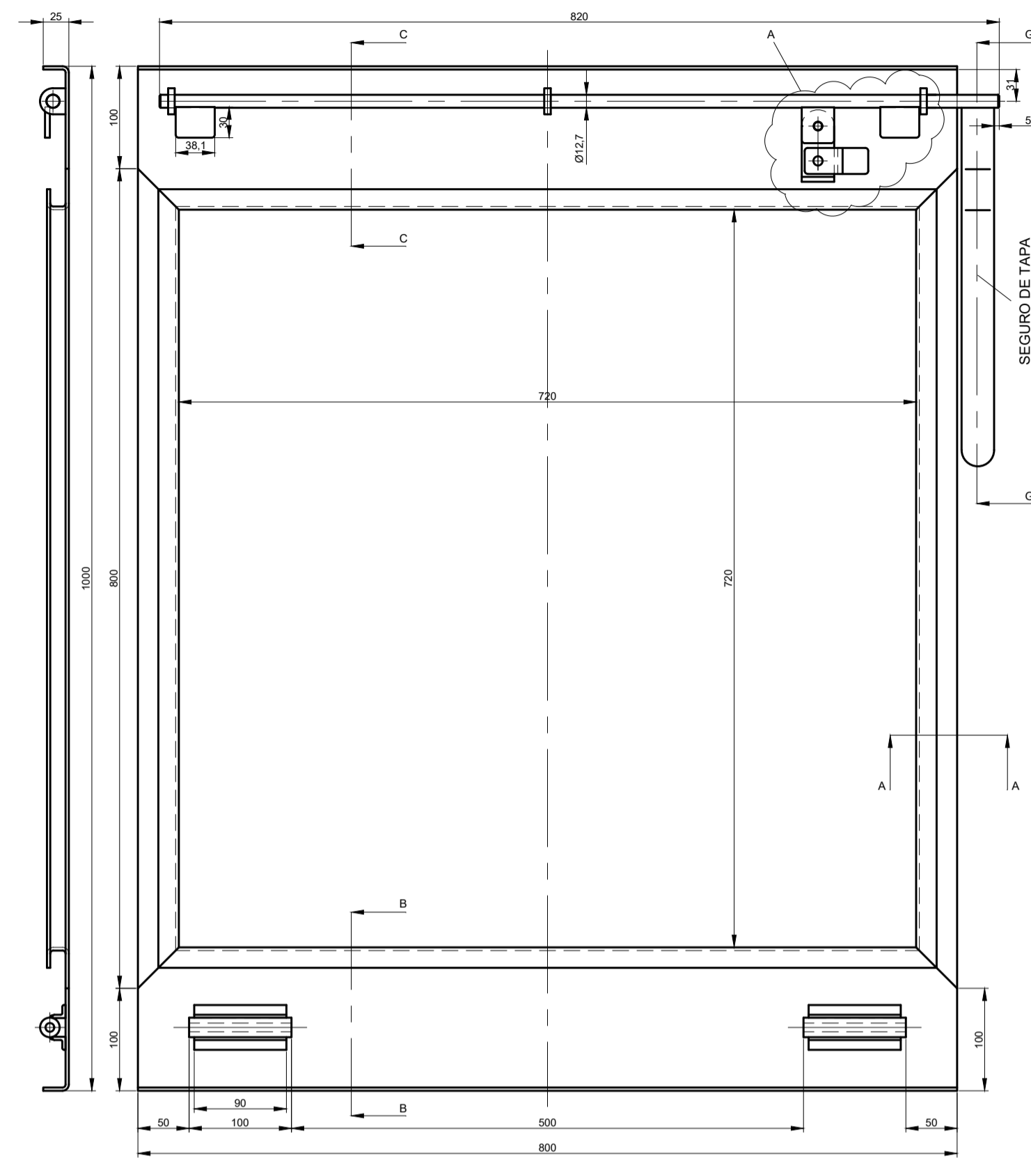
MARCO ESCOTILLA ESCALA: 1:5
